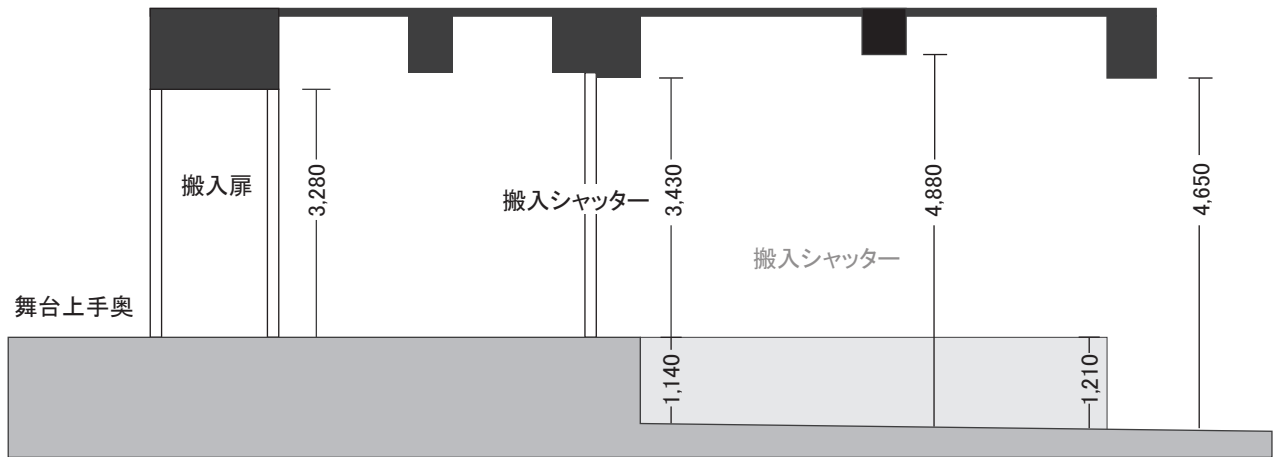
断面図
