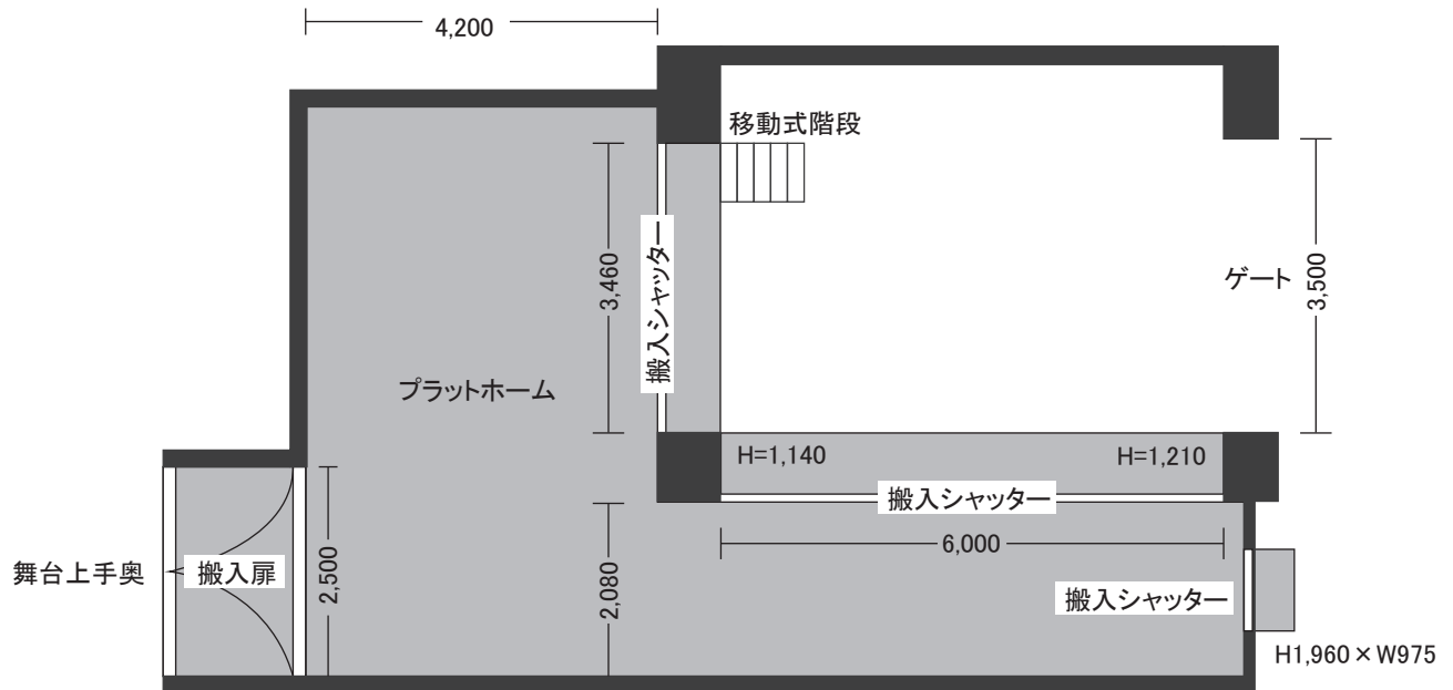
平面図
